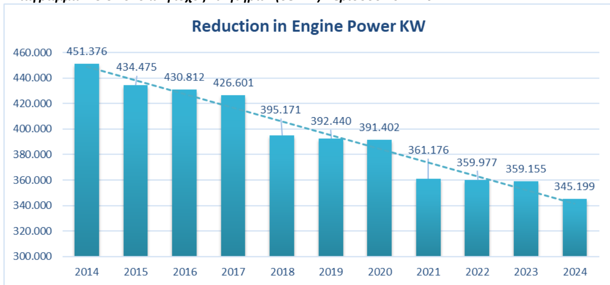
Διάγραμμα Α.3.3 Συνολική ισχύς κινητήρων (σε kW) περιόδου 2014-2024
